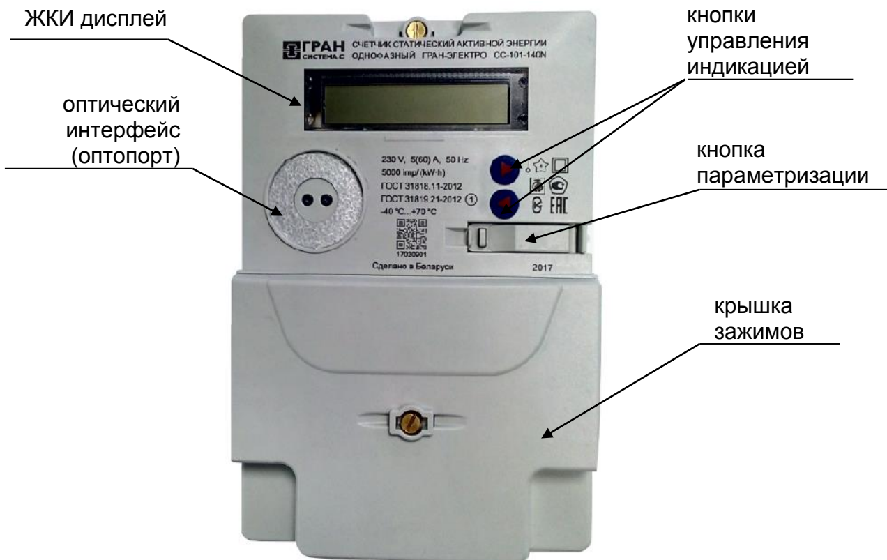
Рисунок 1.2 – Внешний вид счетчика «Гран-Электро СС-101-1X0N»
