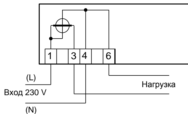
Рисунок Б.1– Подключение счетчиков к однофазной двухпроводной сети 230 В
