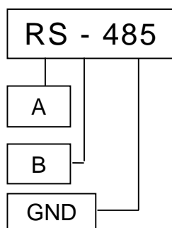
Рисунок Б.2 – Схема подключения счетчика по интерфейсу RS-485
